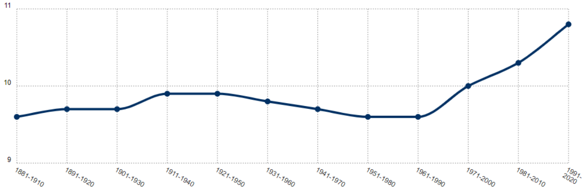
Abbildung 30: Beobachtete Änderung der Lufttemperatur [°C] von 1881-2020 für die Stadt Jülich 38
