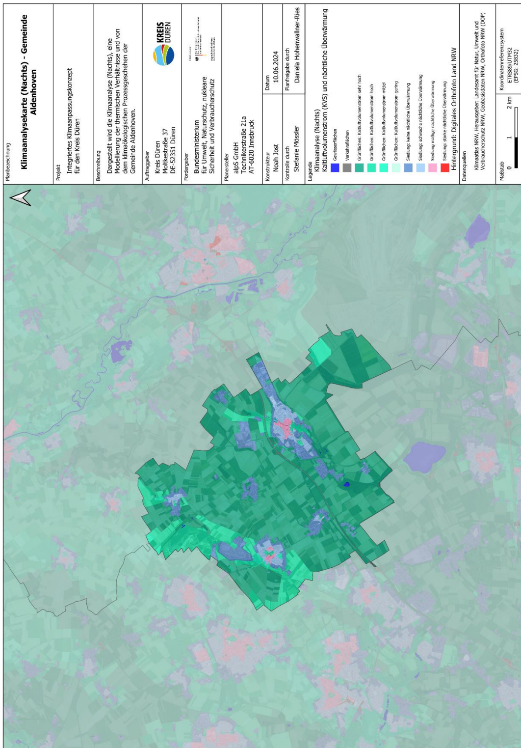
Abbildung 91: Klimaanalyse (Nachts). Dargestellt ist der Kaltluftvolumenstrom und die nächtliche Überwärmung in der Gemeinde Aldenhoven 113 .
