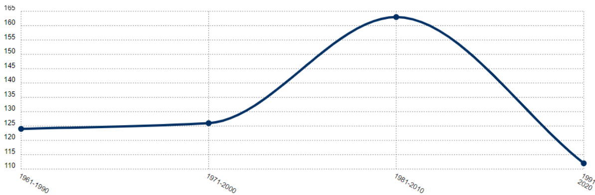
Abbildung 47: Beobachte Änderung der klimatischen Wasserbilanz [mm] von 1961-2020 für die Gemeinde Inden 58
