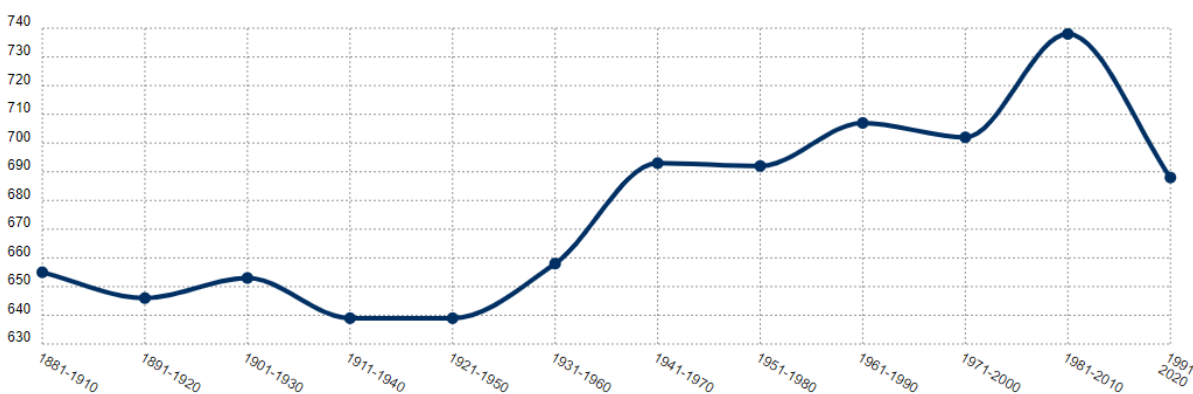
Abbildung 48: Beobachte Änderung der Niederschlagssumme [mm] von 1881-2020 für die Gemeinde Niedezier 59
