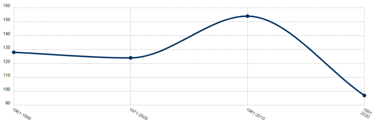
Abbildung 56: Beobachte Änderung der Klimatischen Wasserbilanz [mm] von 1961-2020 für die Stadt Jülich 67
