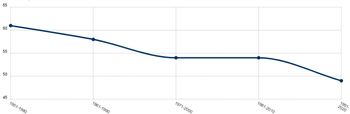
Abbildung 28: Beobachte Änderung der Frosttage [Tage/Jahr] von 1951-2020 für die Landgemeinde Titz 36
