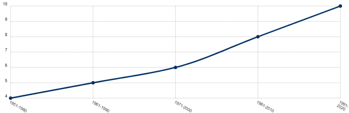
Abbildung 22: Beobachtete Änderung der Heißen Tage [Tage/Jahr] von 1951-2020 für die Gemeinde Niederzier 30
