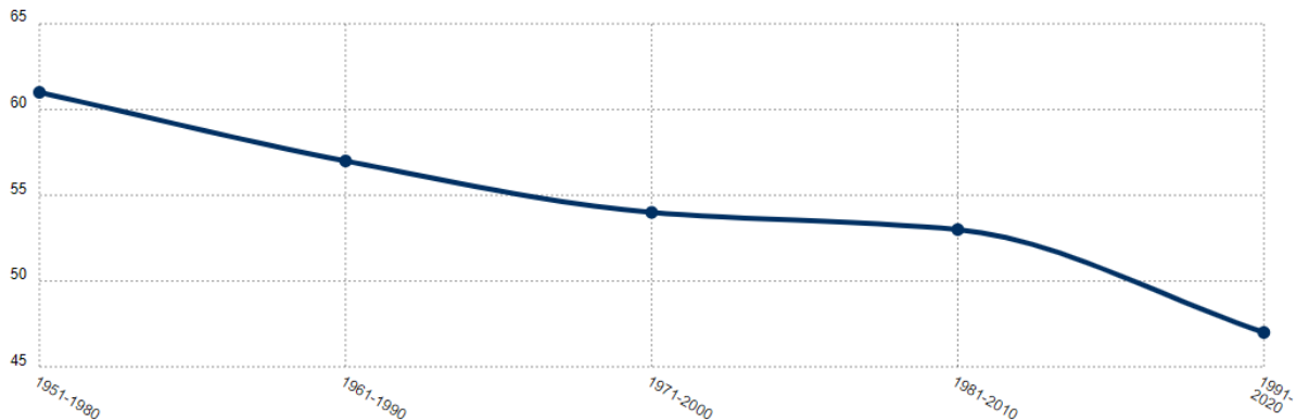
Abbildung 18: Beobachtete Änderung der Frosttage [Tage/Jahr] von 1951-2020 für die Gemeinde Inden 26
