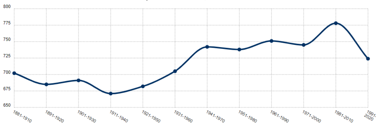
Abbildung 40: Dargestellt ist die Niederschlagssumme in mm für den Kreis Düren in Klimanormalperioden von 1881-2020.
